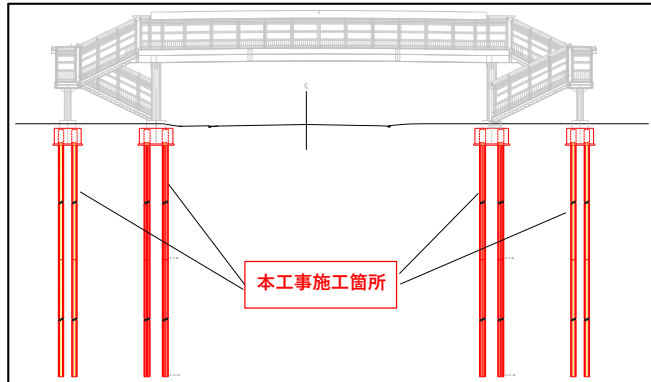
施工箇所側面図
